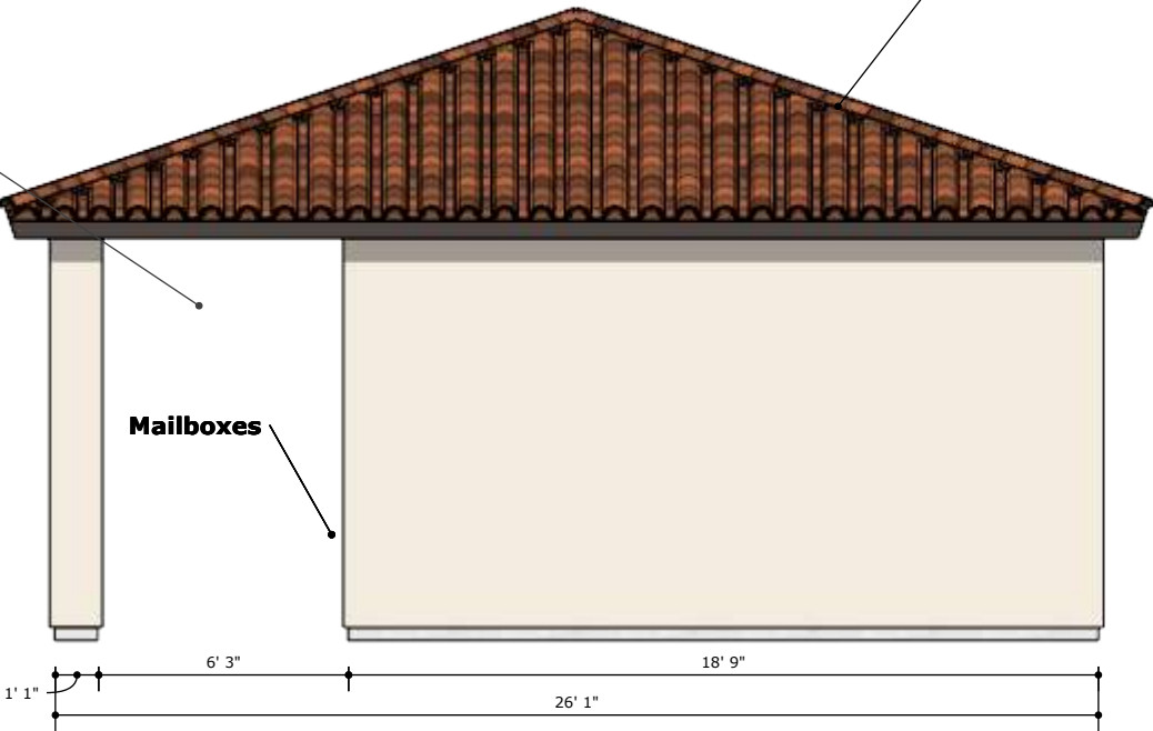
RIGHT ELEVATION
